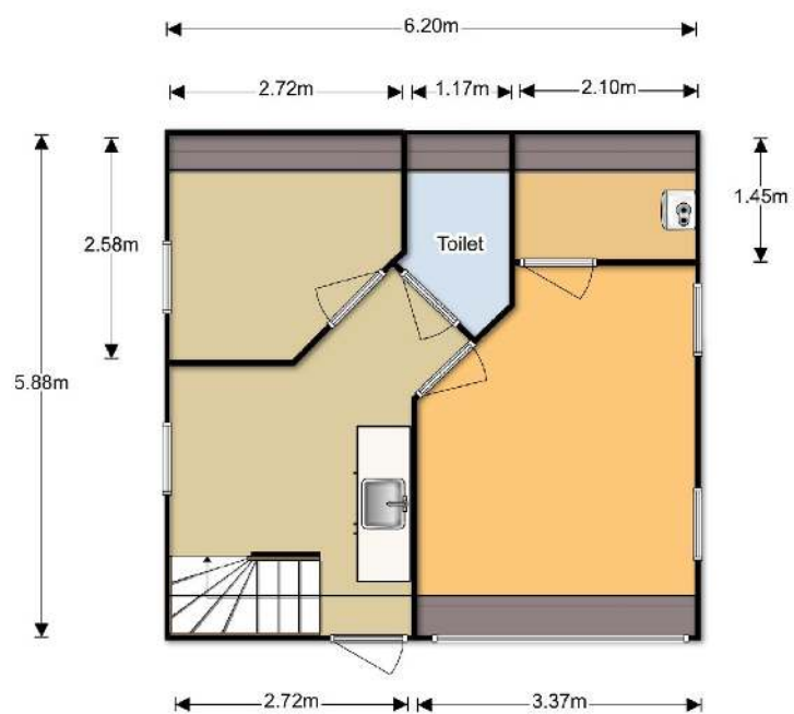
Garage 1e Verdieping
